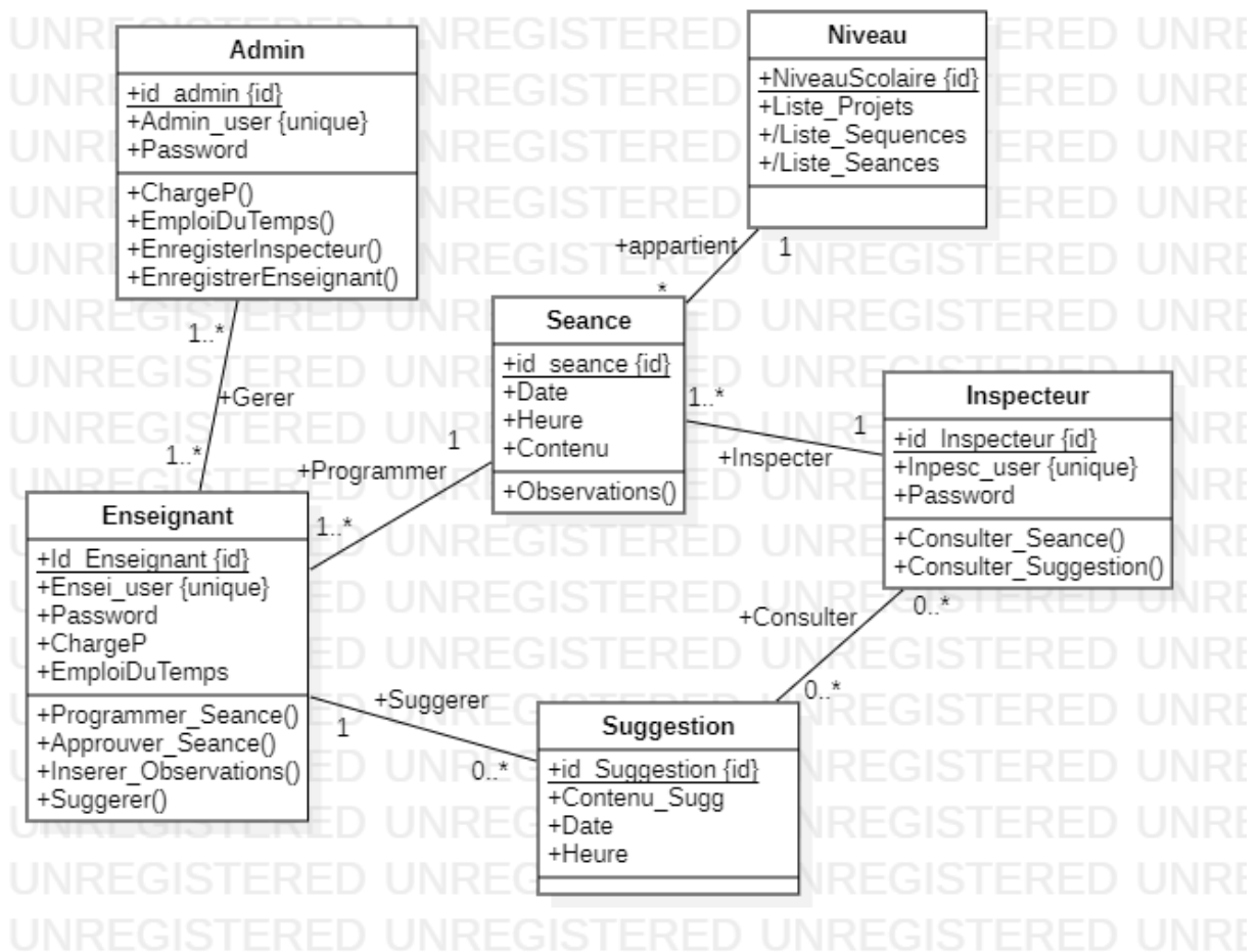
Figure 08. Diagramme de classes
