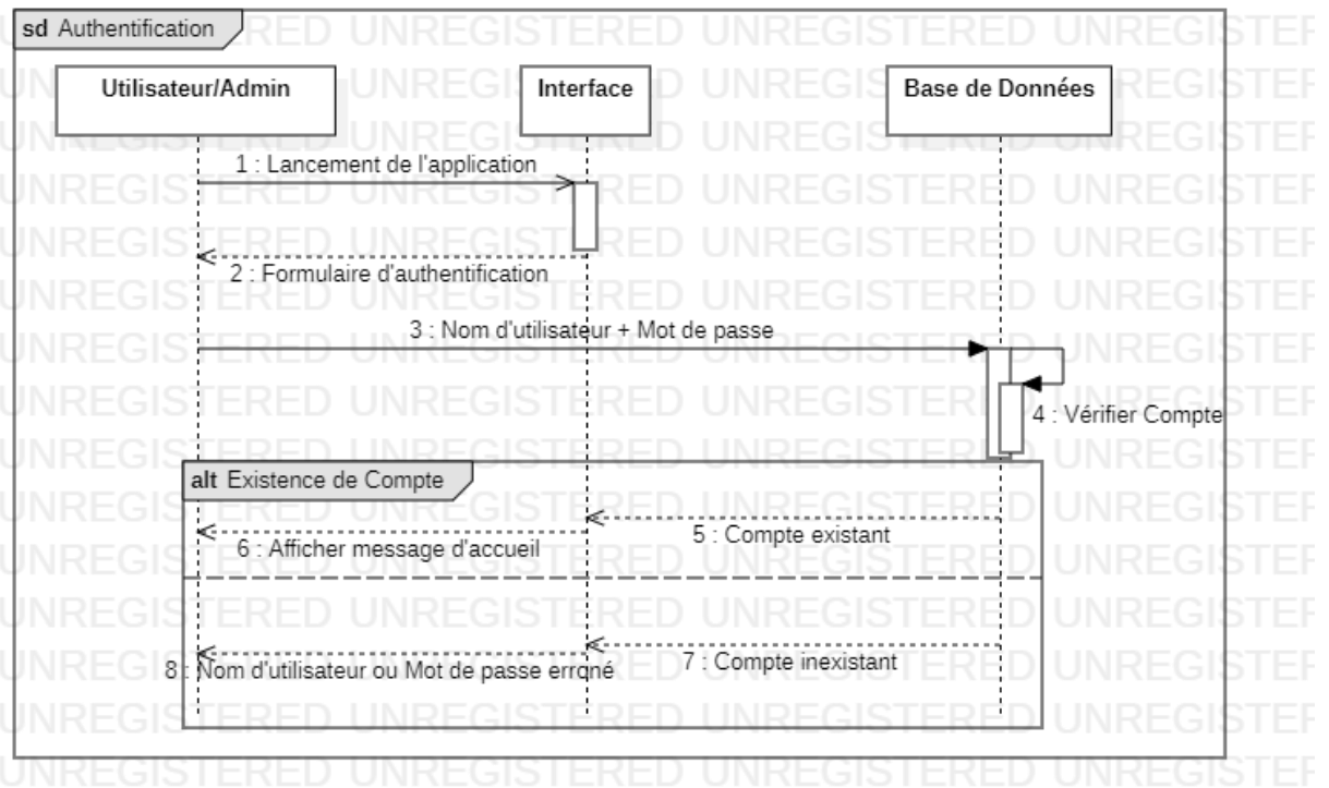
Figure 09. Diagramme Séquence "Authentication"
