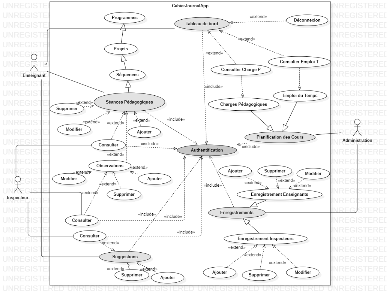
Figure 07. Diagramme de cas d'utilisation
