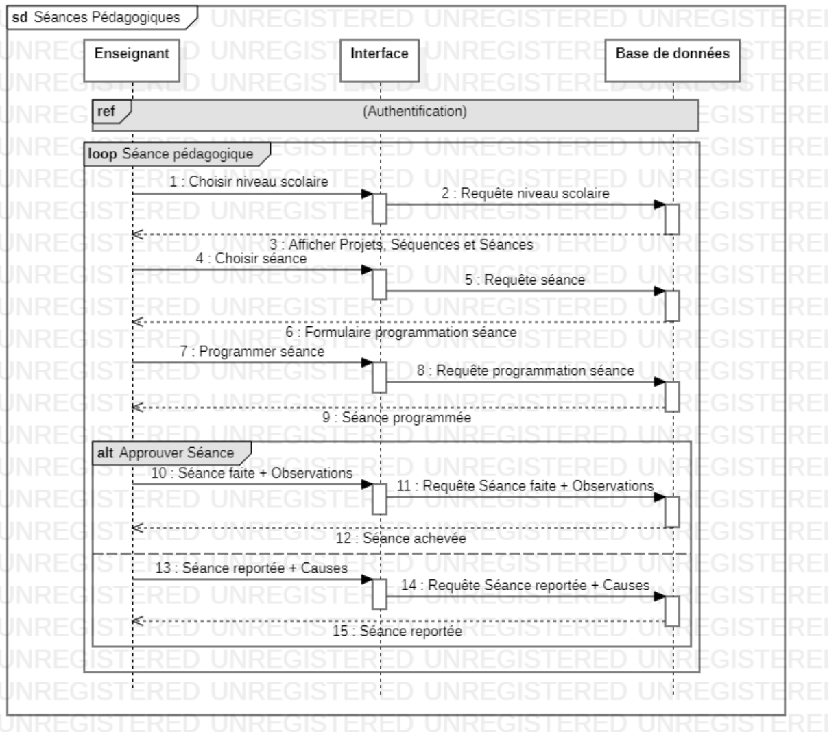
Figure 11. Diagramme Séquence " Séances Pédagogiques"
