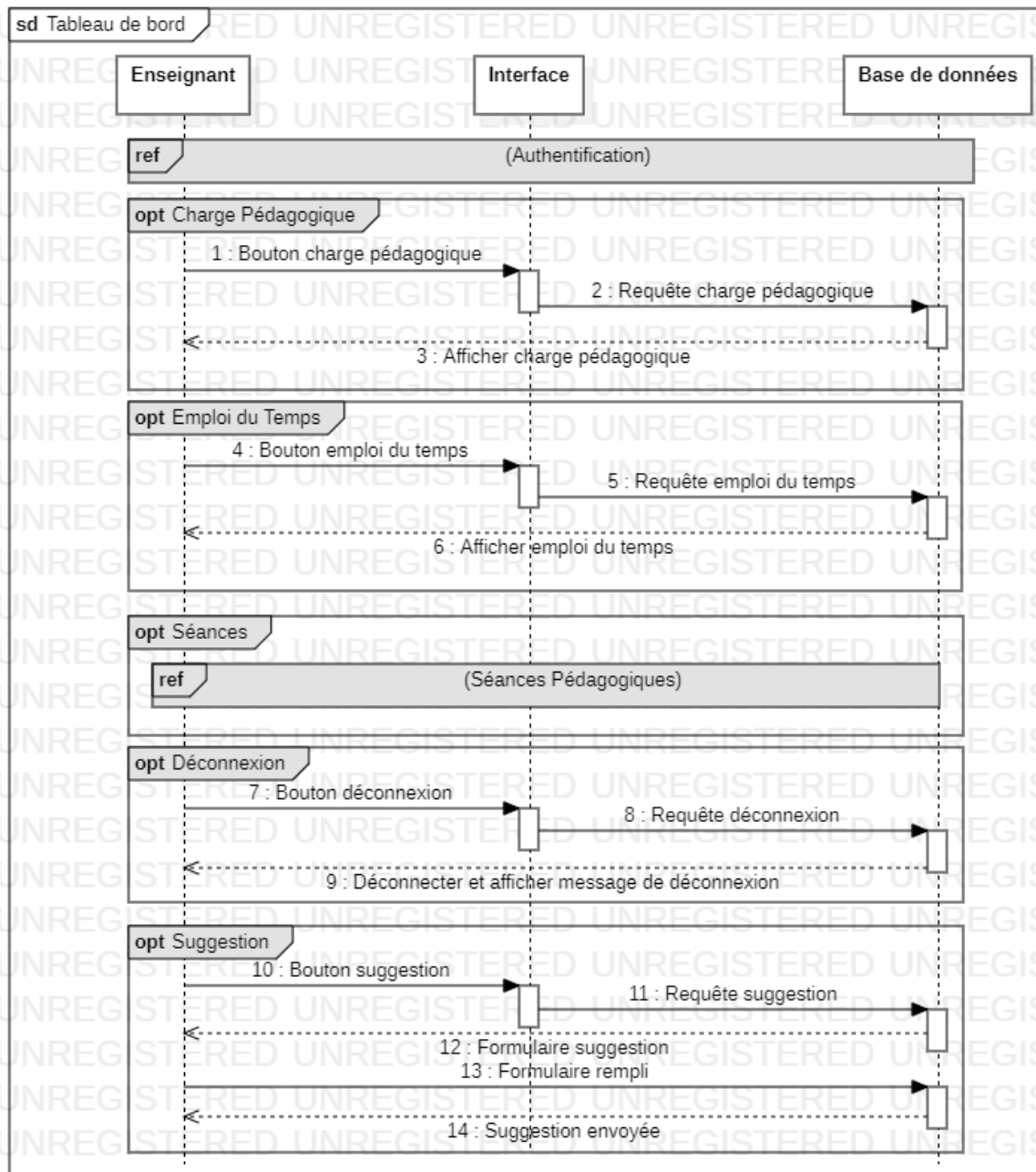
Figure 12. Diagramme Séquence " Tableau de bord "
