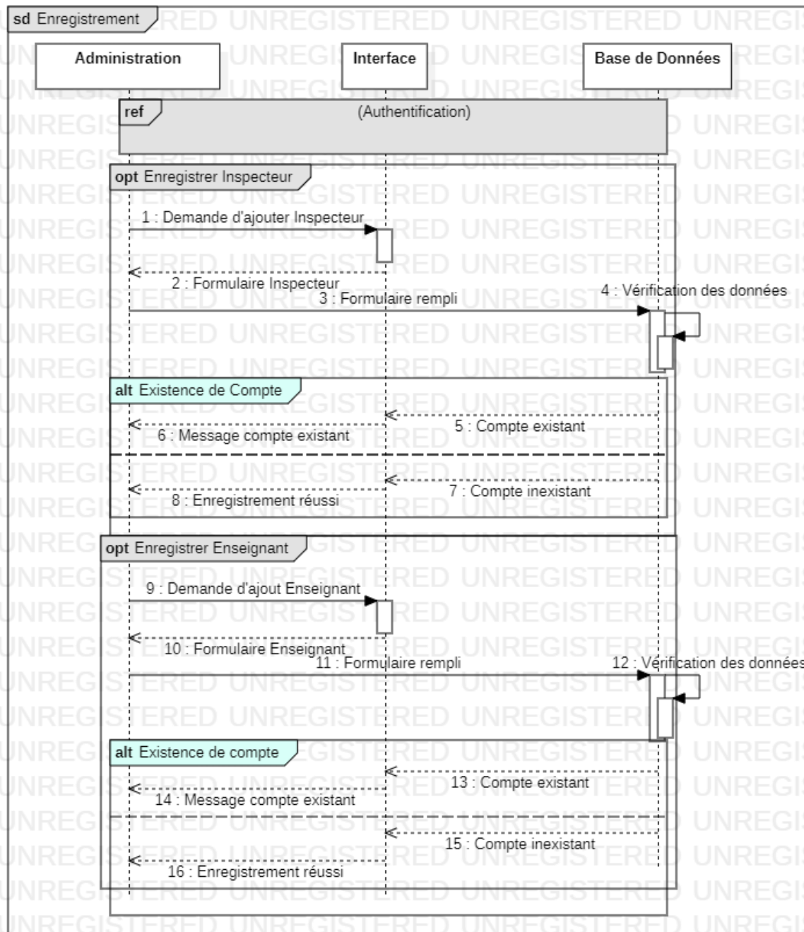
Figure 10. Diagramme Séquence "Enregistrement "
